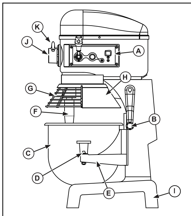
Figura 2. Miscelatore da 22 l e da 33 l, funzioni e comandi.
