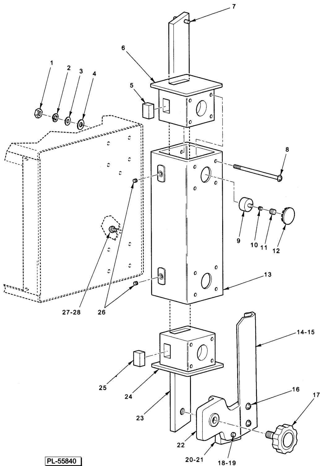
UPPER GUIDE UNIT
