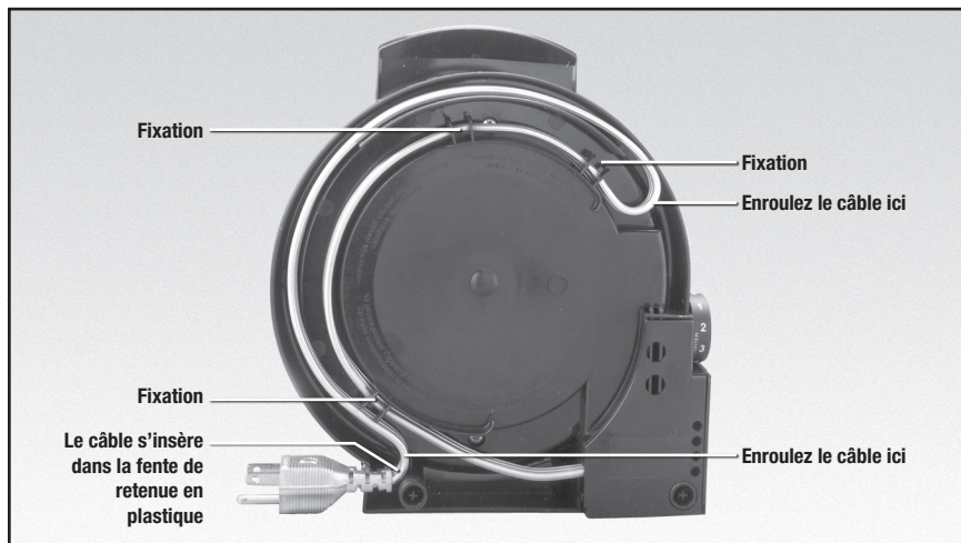
Figure 7. Fixations pour le câble sous la base. Le WaffleCone Express™ se range debout comme illustré.
