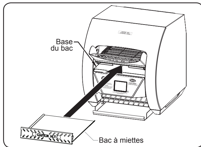
Installation du bac à miettes
