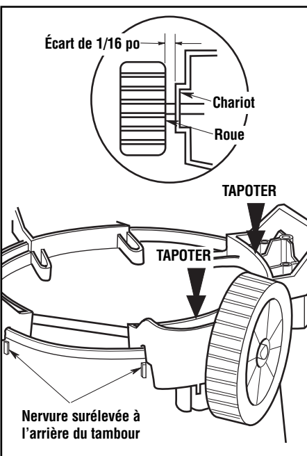
ASSEMBLAGE DU CHARIOT
