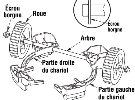
ASSEMBLAGE DU CHARIOT
